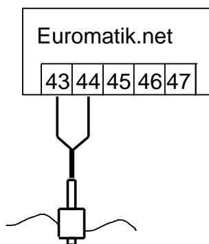
Schwimmerschalter
